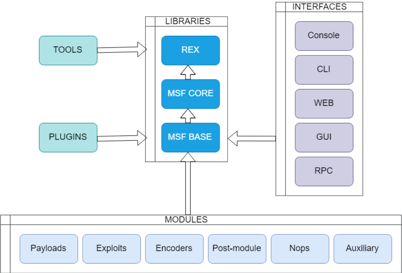
Рисунок 1.2 Структура Metasploit
