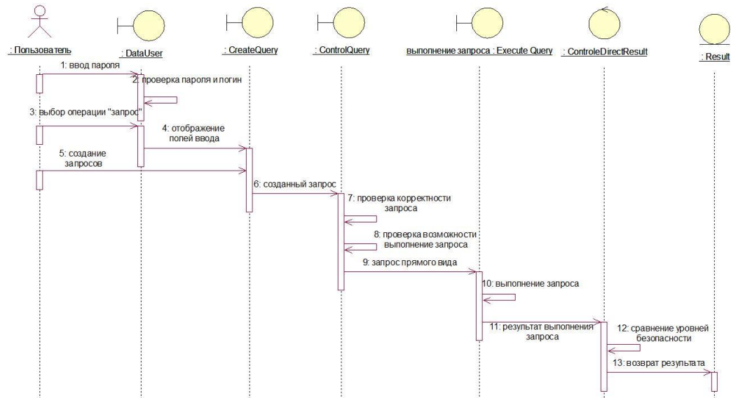
Рисунок 3.4 - Діаграма діяльності процесу контролю прямого запиту користувачів в програмі SecSWD
