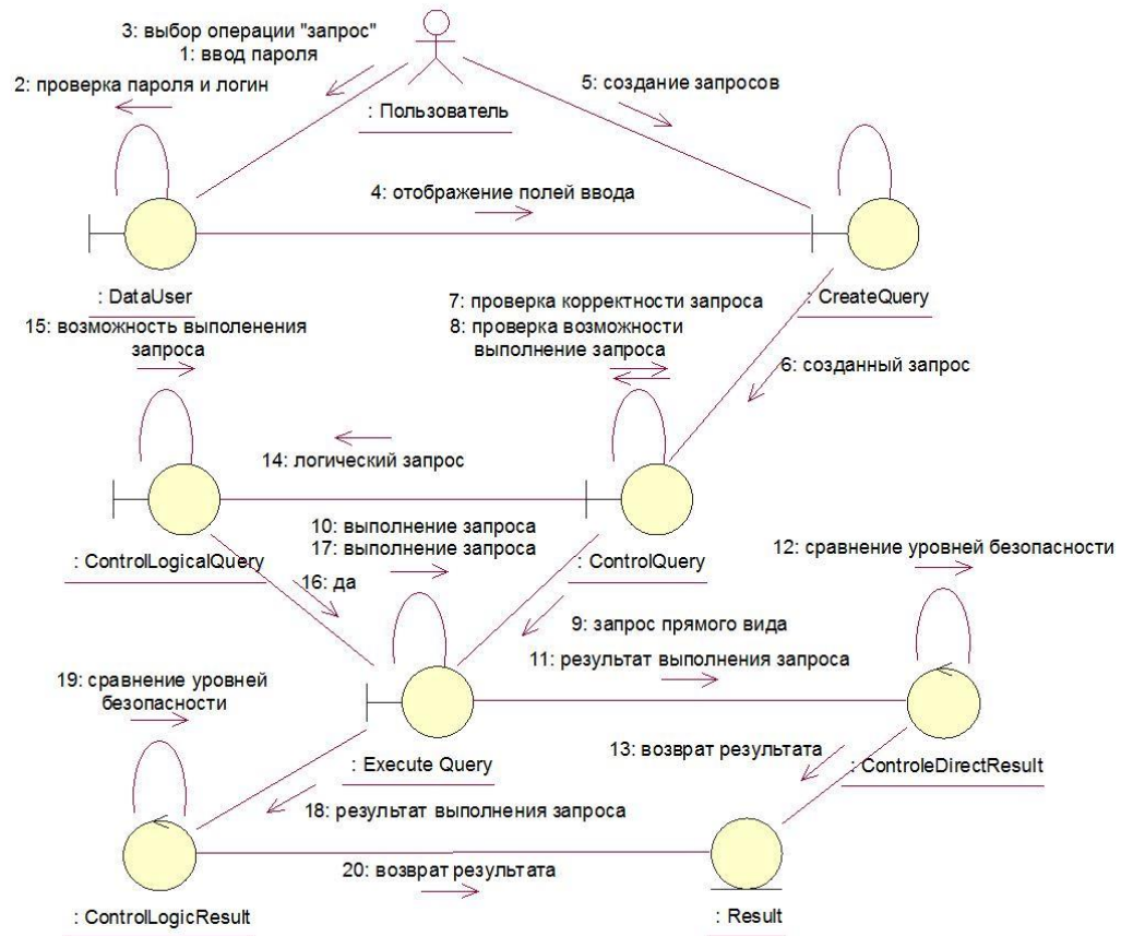
Рисунок 3.6 - Диаграмма кооперативного процесса контроля логических запросов пользователей в программе ContrLSD
