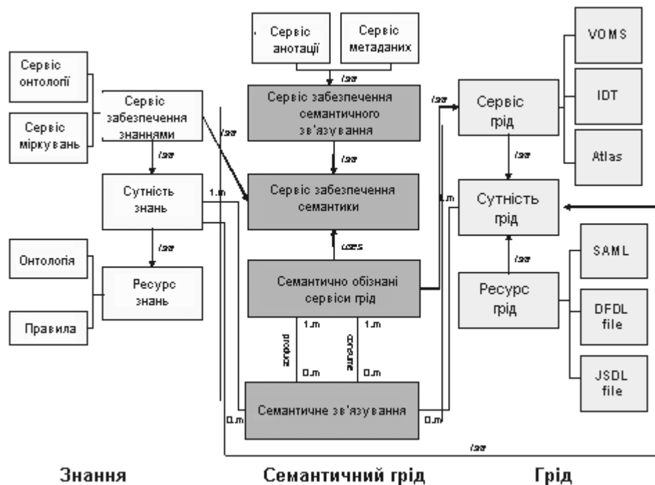
Рисунок 1.15 - Сервіси забезпечення семантики
