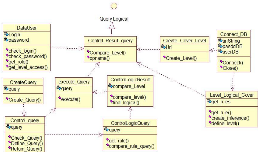
Рисунок 3.5 - Діаграма класів інтерфейсу Query Logical програми ContrLSD
