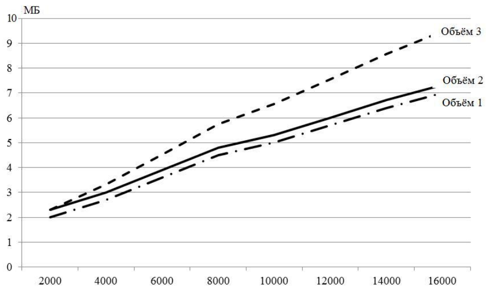
Рисунок 3.13 - Діаграма залежності обсягів простору зберігання даних від кількості триплетів
